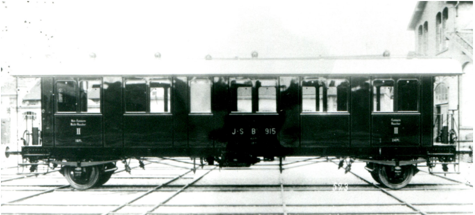
Ablieferungszustand des B 3505 von 1902 (Foto: SIG)
